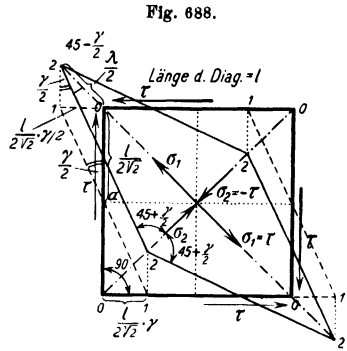
Verformung eines Teilchens durch Schubspannungen.
