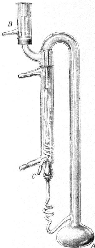
Diffusionspumpe nach Volmer.
