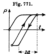
Hysteresis-Schleife nach Prandtl.
