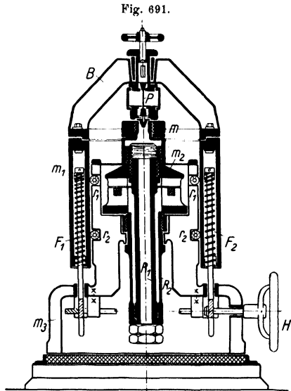
Dynamische Materialprüfmaschine der Firma C. Schenk-Darmstadt.
