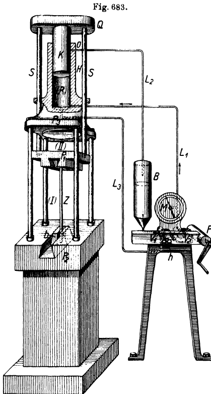
Festigkeitsprüfmaschine der Firma Amsler & Co., Schaffhausen.
