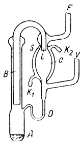
Diffusionspumpe nach Langmuir.
