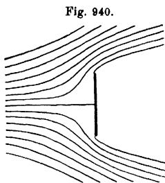
Fig. 940. Kirchhoffsche Strömung an einer ebenen Platte.
