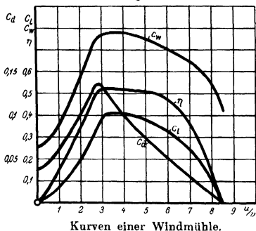
Kurven einer Windmühle.
