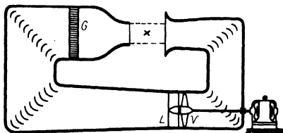
Windkanalanordnungen.
