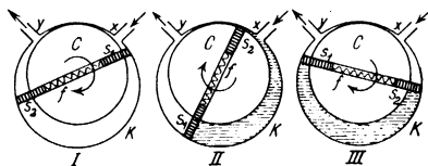
Schematische Darstellung der Wirkungsweise einer Kapselpumpe.
