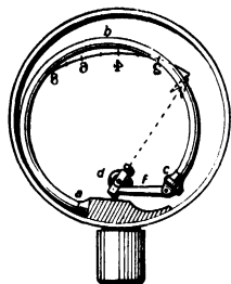
Röhrenfederanometer.
