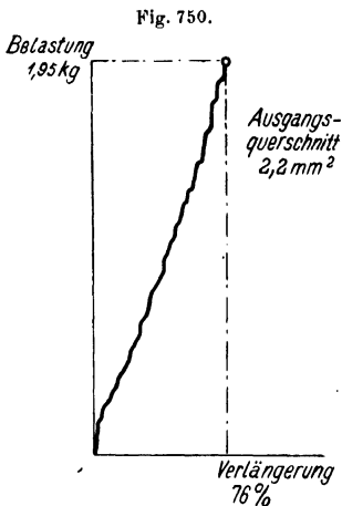
Zug-Dehnungsdiagramm für Zink-Einkristalldraht.
