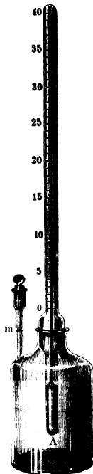
Pyknometer für feste Körper und Flüssigkeiten.
