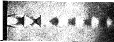
Wellen mit ausfließender Druckluft.
