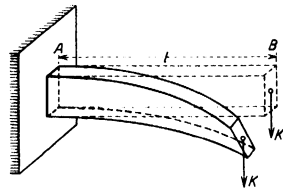
Kippung eines hochkantig gestellten Balkens.
