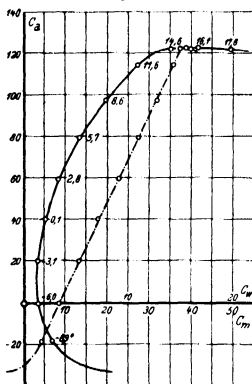
Polarkurve (ausgezogen) und Momentenkurve (strichpunktiert). Die Zahlen sind das Hundertfache von \alpha , c_w und c_m .
