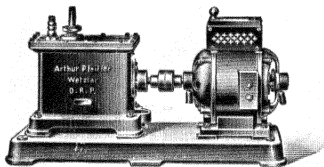
Rotierende Ölluftpumpe nach Pfeiffer.
