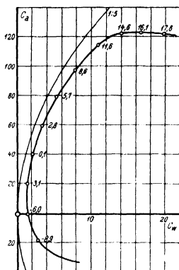
Parabel des induzierten Widerstandes.
