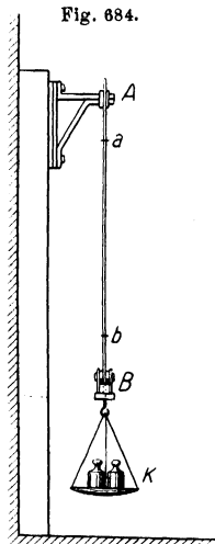
Fig. 684. Prüfung der Dehnung und Festigkeit von Drähten und dünnen Stäben.
