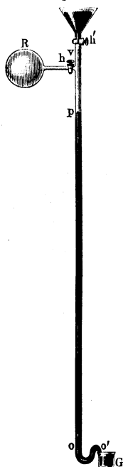
Schema einer Quecksilber- pumpe nach Sprengel.
