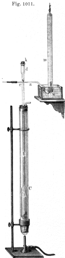
Dampfdichte nach Victor Meyer.
