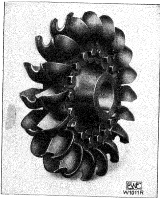
Pelton-Rad.
