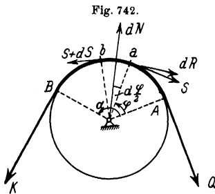
Fig. 742. Kräfte am Seil über einer rauen Walze.
