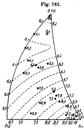
Verteilung der Höchstlasten beim Doppelgleiten von Al als Funktion der Anfangslage der Drehachse (nach v. Göler u. Sachs).
