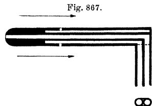
Fig. 867. Staurohr nach Prandtl.
