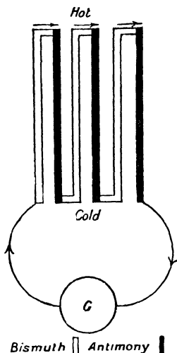
FIG. 128.—Thermopile.
