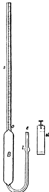
FIG. 26.—Dilatometer.
