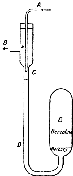
FIG. 8.—Thermostat.
