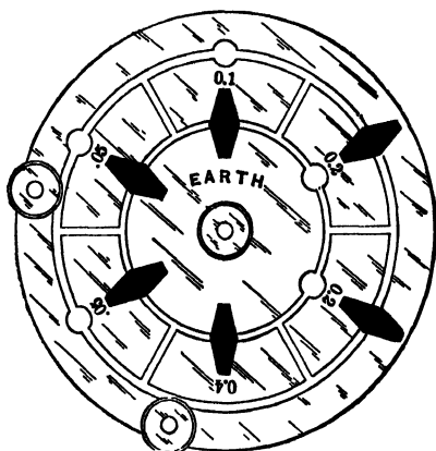
Fig. 83.—Standard Microfarad Condenser.
