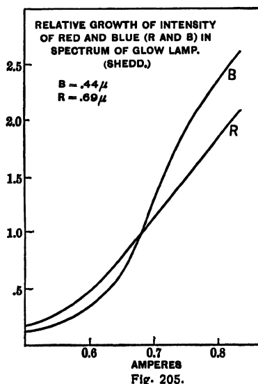
Fig. 205.
