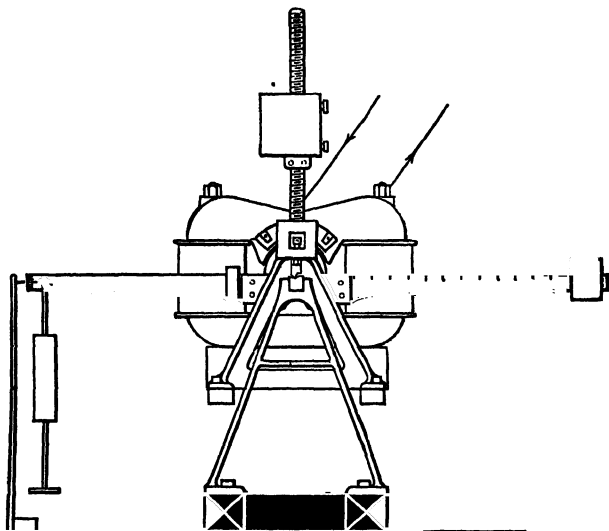
Fig. 19. — Brackett Cradle Dynamometer.
