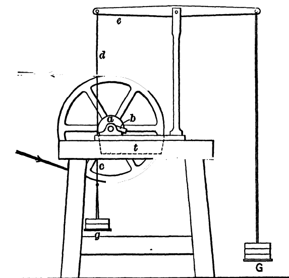
Fig. 20. — Raffard Dynamometer.
