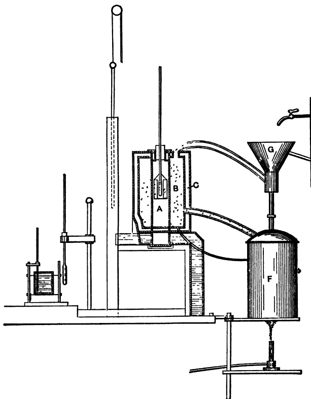
Fig. 130. — Regnault's Apparatus.
