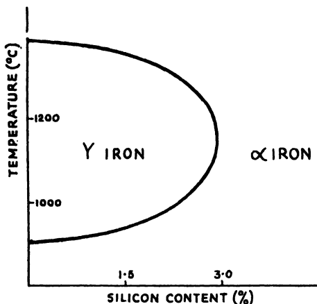
FIG. III-1.—IRON-SILICON DIAGRAM.
