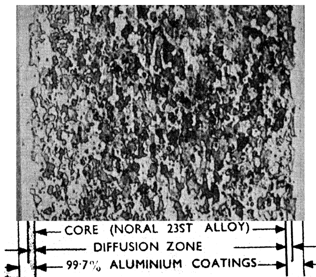
FIG. VII-3.—“CLAD” ALUMINIUM COMPOSITE PLATE.
