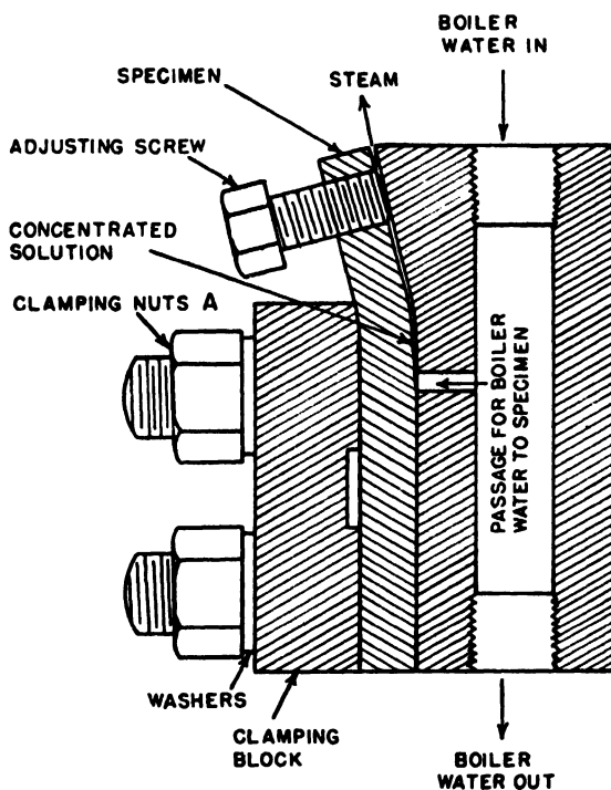
FIG. IV-13.—EMBRITTEMENT DETECTOR.
