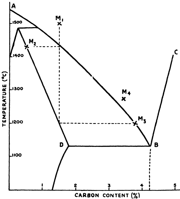
FIG. III-4.—AUSTENITE REGIONS-(Fe-C) DIAGRAM.
