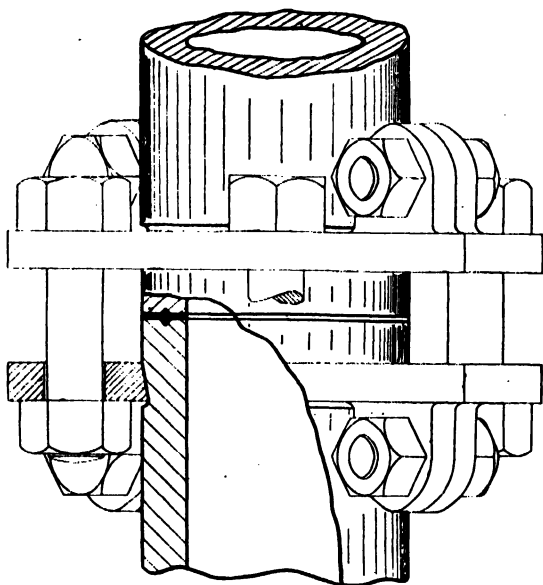
FIG. XIX-3.—JOINT FOR KEREKUSH PIPE.
