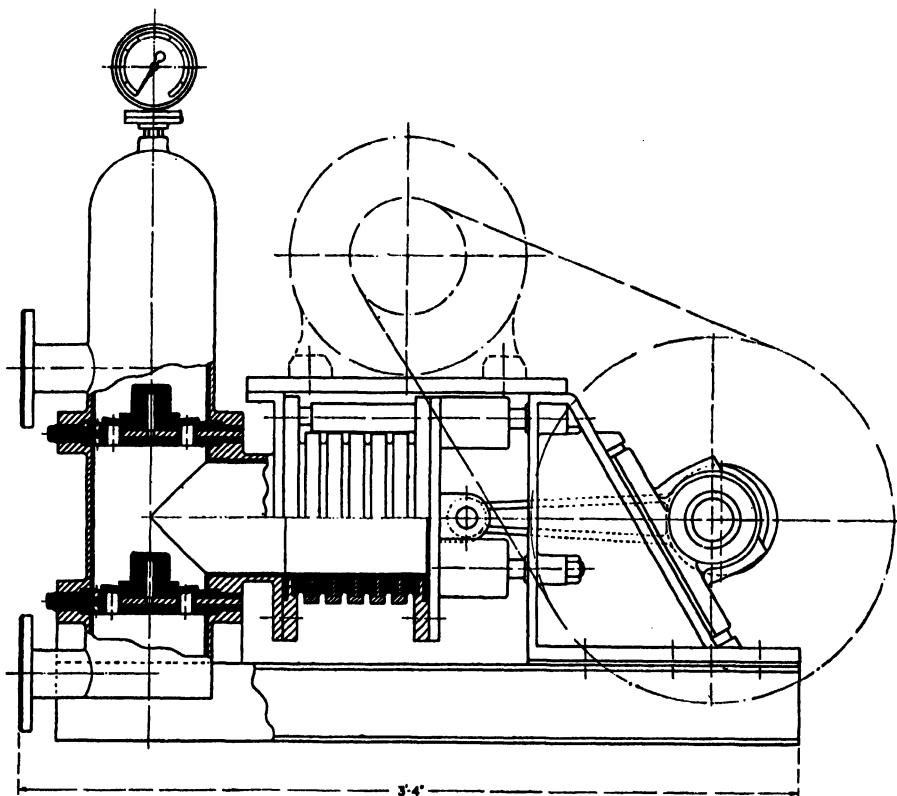
FIG. XIX-14.—THE PERISTALTIC PUMP.
