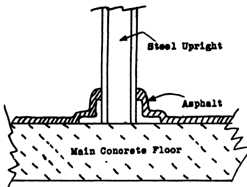
FIG. XIV-1.—ASPHALT FLOOR PROTECTION.
