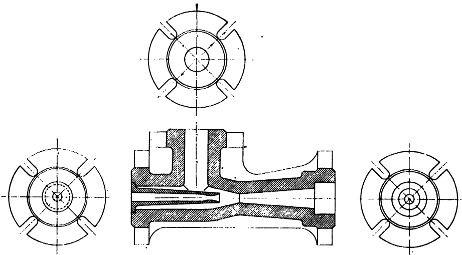
FIG. X-3.—SILICON-IRON EJECTOR.
