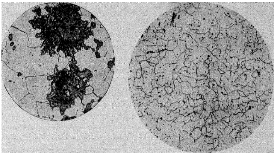
FIG. III-18b.—WHITEHEART MALLEABLE CAST IRON.
