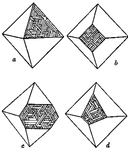
Abb. 71. Form der Widmannstetter'schen Figuren in Abhängigkeit von der Schnittlage. a = Schnitt // einer Oktaederfläche; b = Schnitt // einer Würfel- fläche; c = Schnitt // einer Rhomben- dodekaederfläche; d = beliebige Schnittlage. (Nach Tschermak, Lehrbuch der Mineralogie. 1894.)
