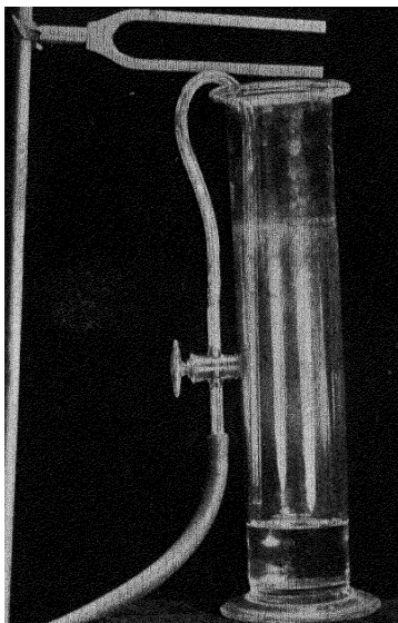
A. Tuning fork over jar.
