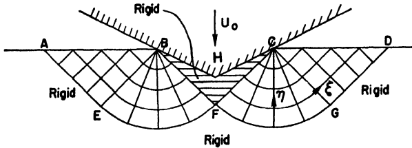
FIG. 27. Straight sided indenter.
